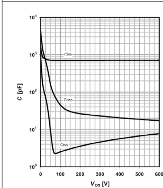
Typ. capacitances
