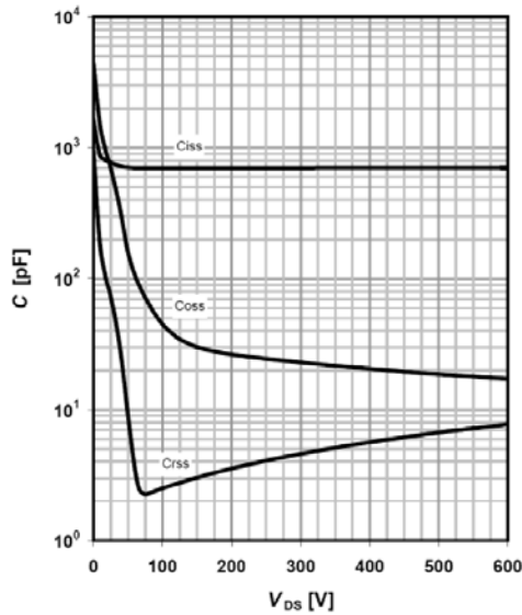
Typ. capacitances
